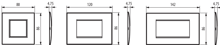
LNC4802...
