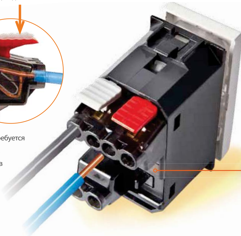
Жесткий и гибкий кабель: зачистка изоляции - 12 мм
