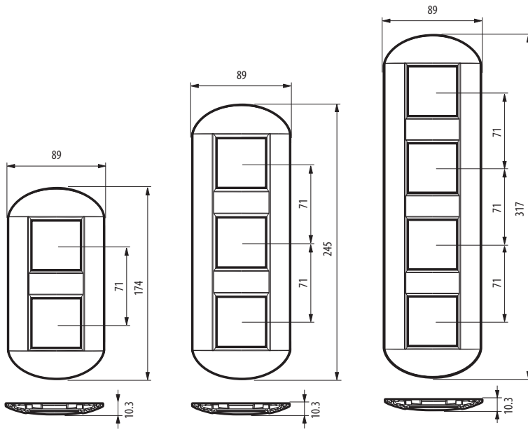
LNB4802M2...
