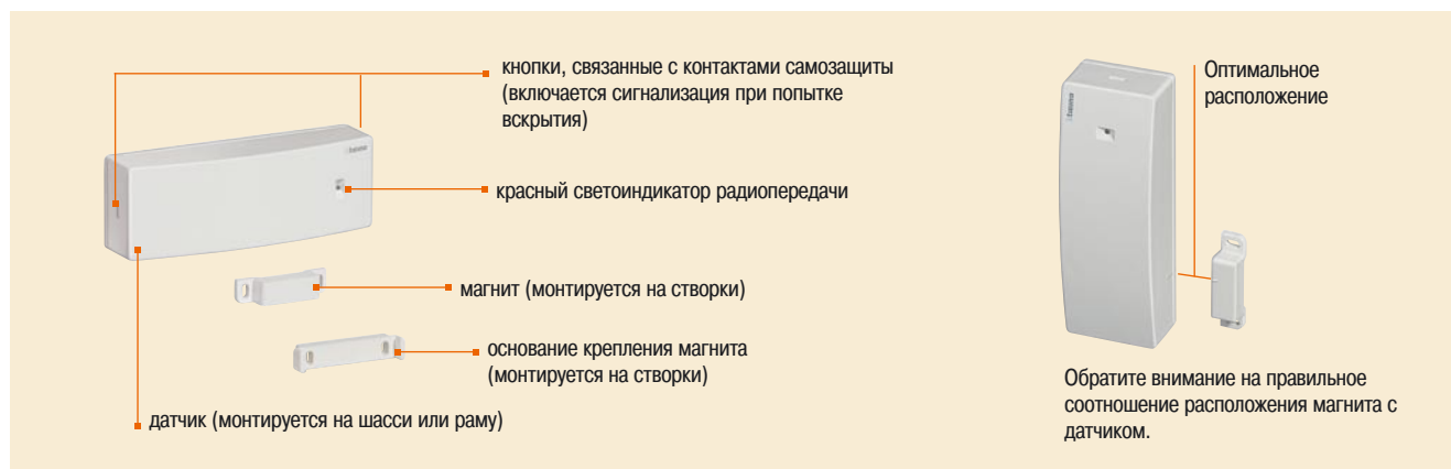
установка магнитного датчика на окне
